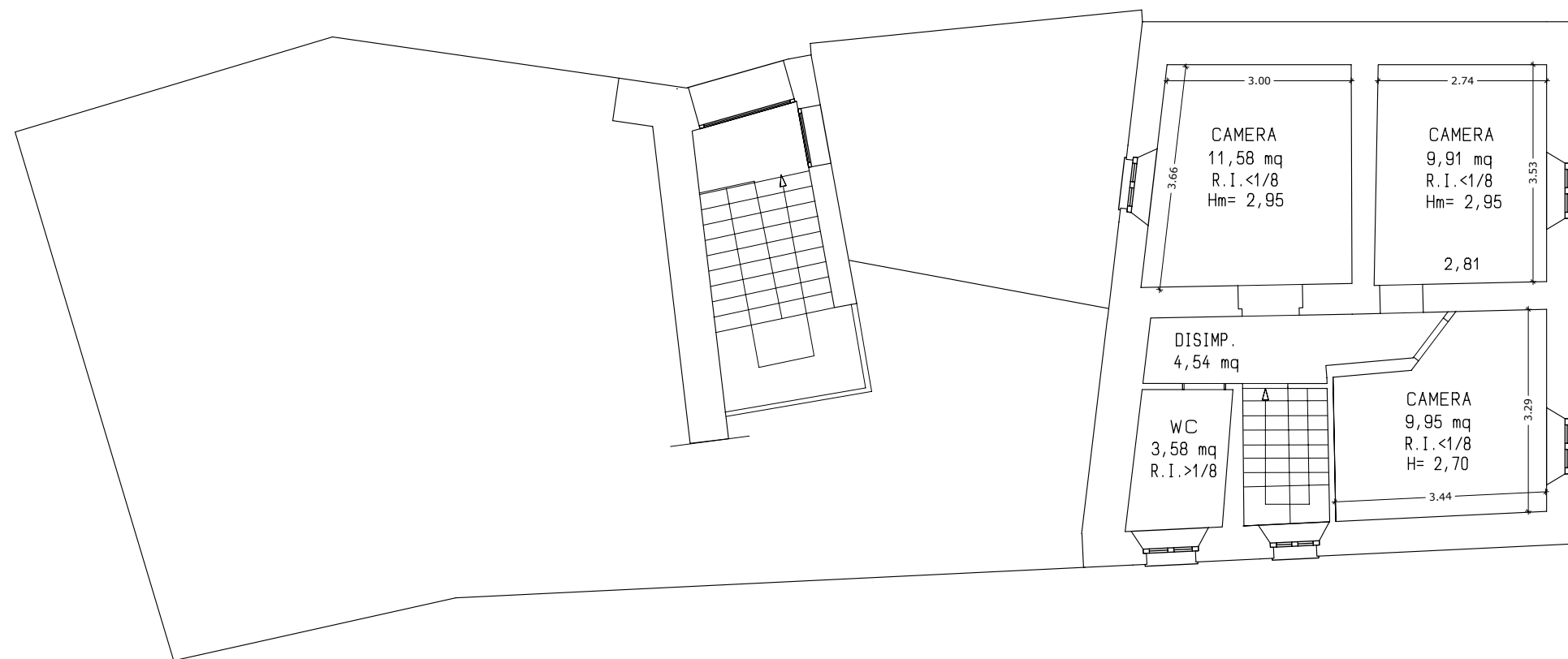
PIANO SECONDO
